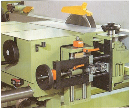
Εικ. 7.3 Δισκοπρίονο
