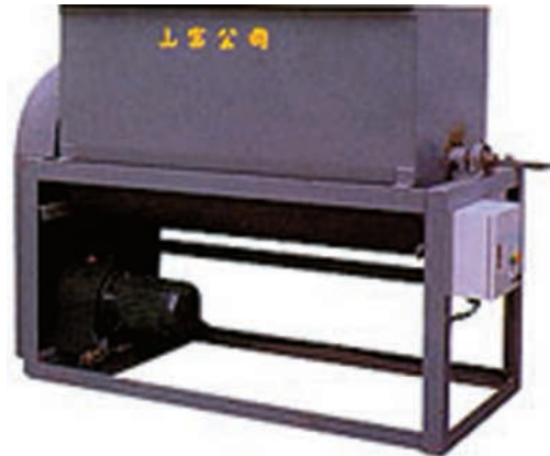
Εικ. 11.5 Μηχανή ανάμειξης ξυλοτεμαχιδίων με συγκολλητική ουσία
