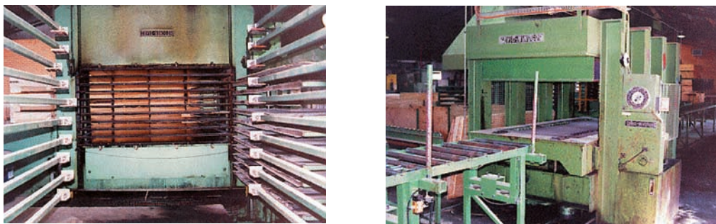
Εικ. 10.7 Πρέσες για παραγωγή ξυλοφύλλων
