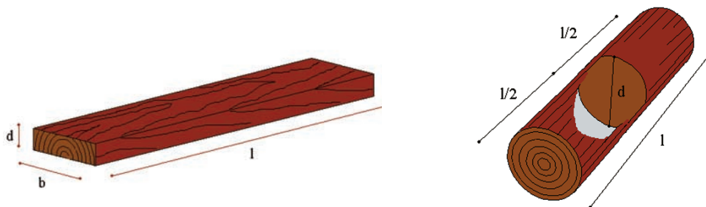
Σχ. 14.1 Ογκομέτρηση μασίφ πριστής ξυλείας Σχ. 14.2 Ογκομέτρηση μασίφ στρογγύλης ξυλείας
