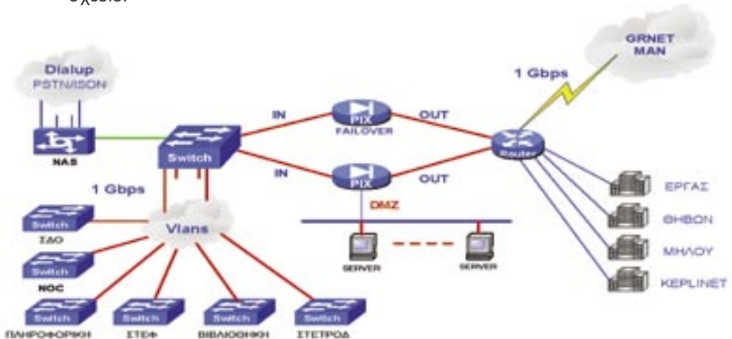
Δίκτυο Κορμού Gigabit Ethernet του TEI Αθήνας
